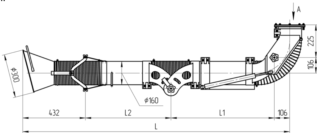
Монтажный кронштейн (поз.13 рис.3.1)
