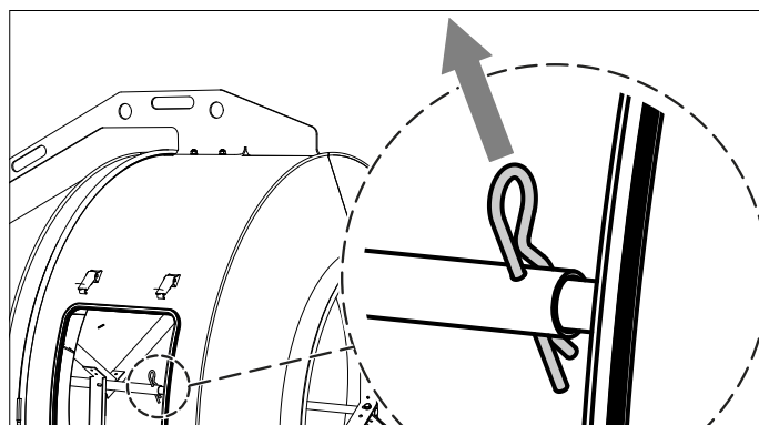
Рис. 5.2: Шплинт
