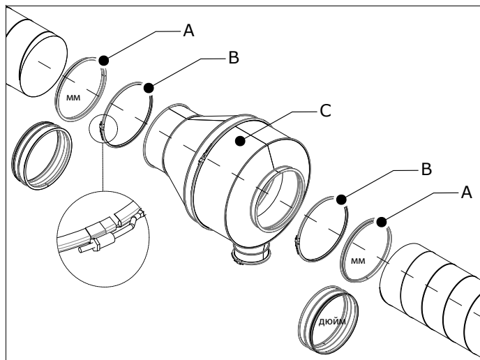
Рис. 4.1: Установка искрогасителя
