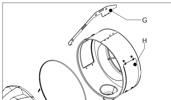
Рис. 2.1: Основные части
