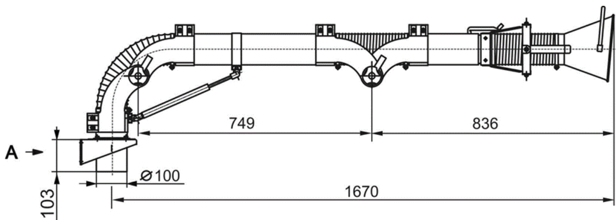
Модификация для вертикальной установки DELI-100-15-S
