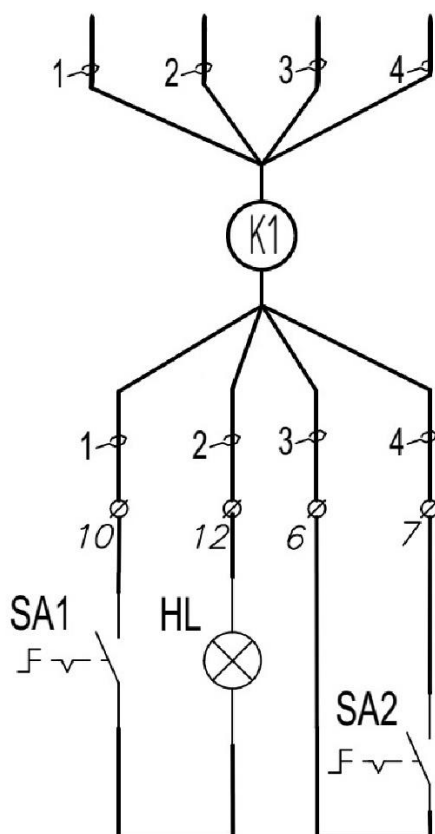
Рисунок Г.1 – Схема подключения устройства с установкой под опорой (H)
