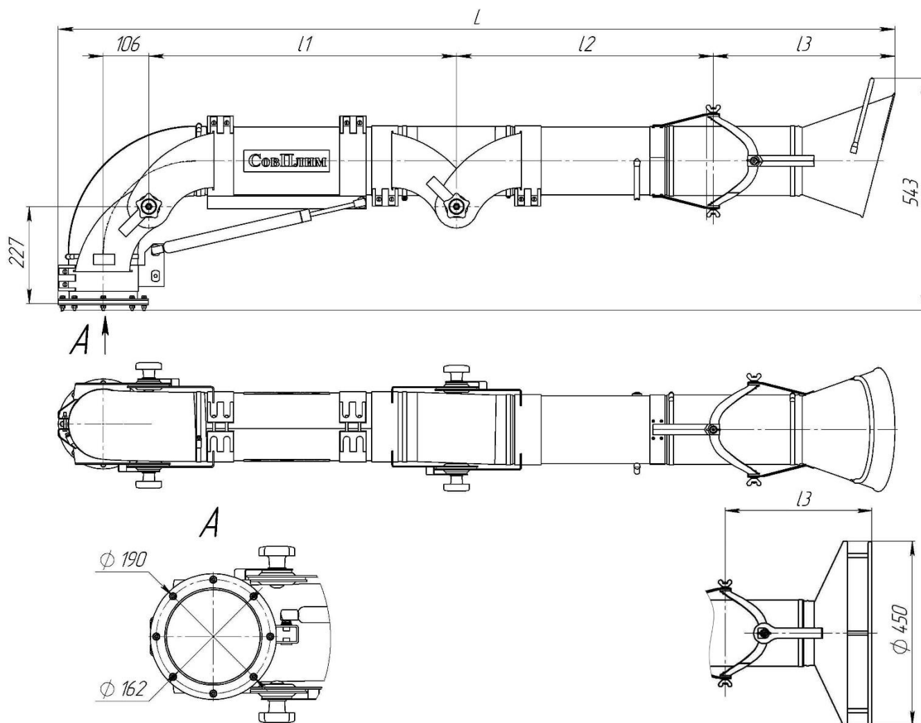
Рисунок А.2 – Габаритные размеры устройства, предназначенного для установки над опорой (S)
